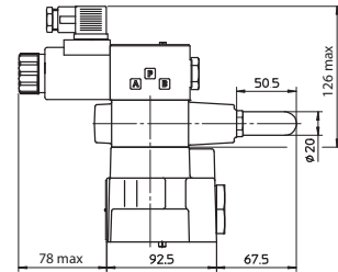
AGIU-10/10/**-E(R)X ; Mass = 5,6 Kg
