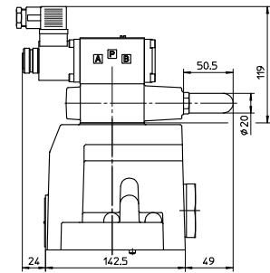
AGIU-32/10/**-IX; Mass = 11,4 Kg
