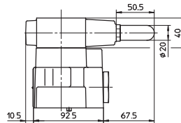
AGIS-10 ; Mass = 3,8 Kg AGISR-10 ; Mass = 4 Kg AGIU-10 ; Mass = 3,8 Kg
