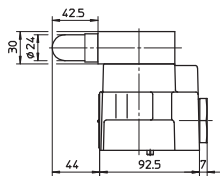
AGIR-10 ; Mass = 3,3 Kg AGIRR-10 ; Mass = 3,5 Kg
