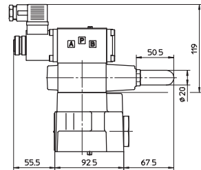
AGIU-10/10/**-IX ; Mass = 5,3 Kg
