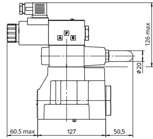
AGIU-20/10/**-E(R)X; Mass = 7,8 Kg
